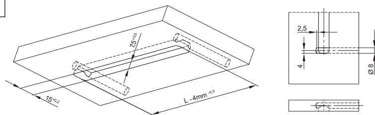
Fräsmaß Kabelausgang hinten Dimensions of milling out, rear cable outlet
