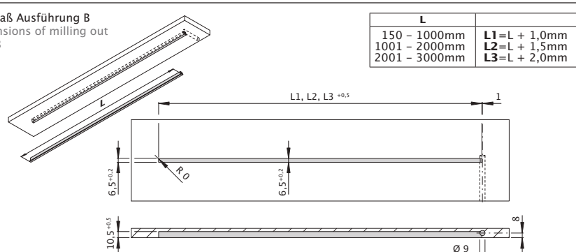
Fräßmaß Ausführung C Dimensions of milling out type C
