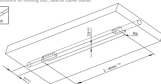
Fräsmäß Kabelausgang seitlich Dimensions of milling out, lateral cable outlet
