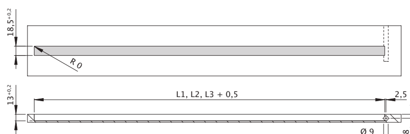
Fräsmaße Dimensions of milling out
