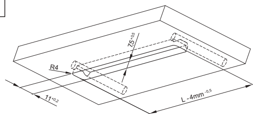
Fräsmäß Kabelausgang hinten Dimensions of milling out, rear cable outlet
