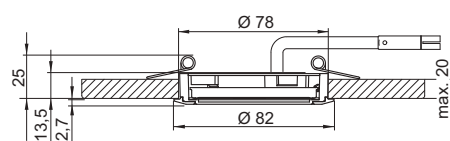
Deckeneinbauleuchte Downlight
