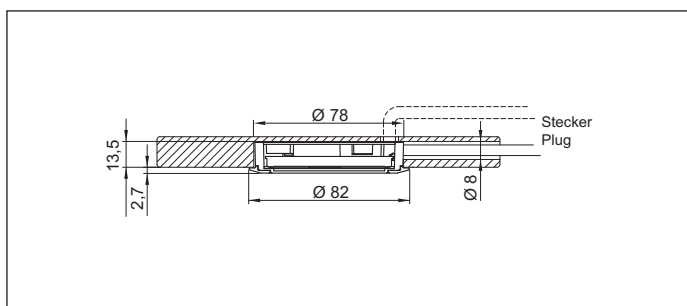
Deckeneinbauleuchte Downlight
