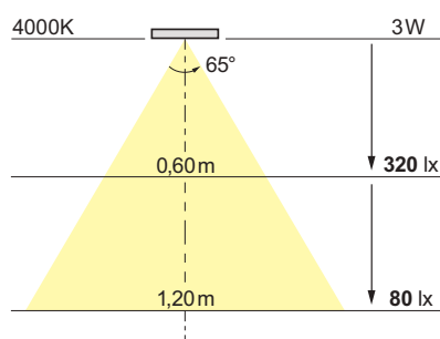
Lichtdiagramm Lighting diagram
