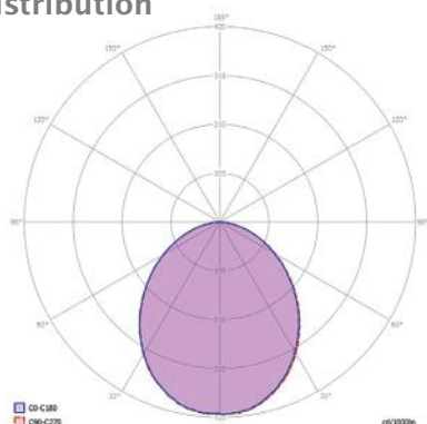
Lichtverteilung Light distribution
