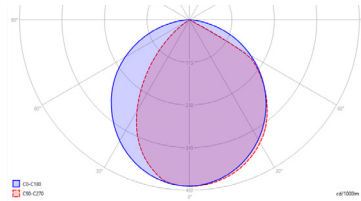
Profil Oben (A)
