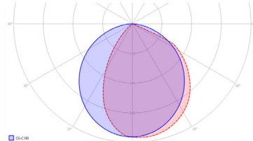
Profil Mitte vertikal (C)
